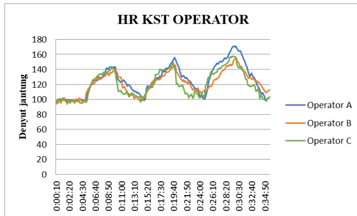
Gambar 2. Grafik hasil pengukuran denyut jantung KST operator [2]
